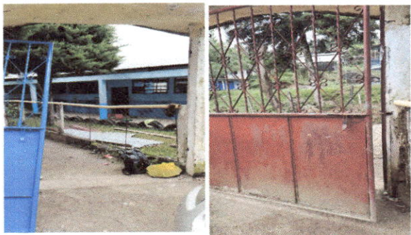
Foto 9: al portón de la entrada, se le cambió la lámina de abajo, se enderezó porque estaba torcido, se mejoraron las bisagras, el lugar del candado y se pinto.
